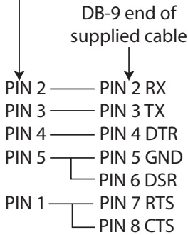
DIN to DB-9 Cable
